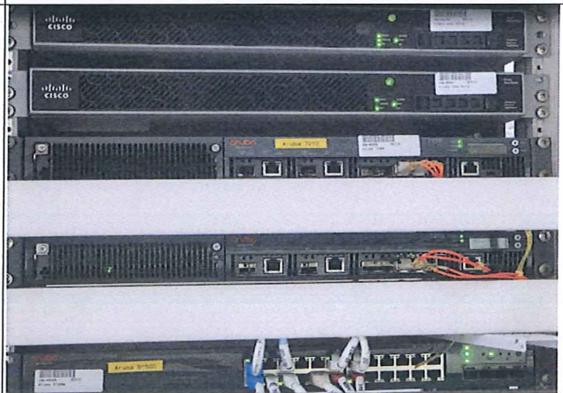
wifi 無線網路設備
